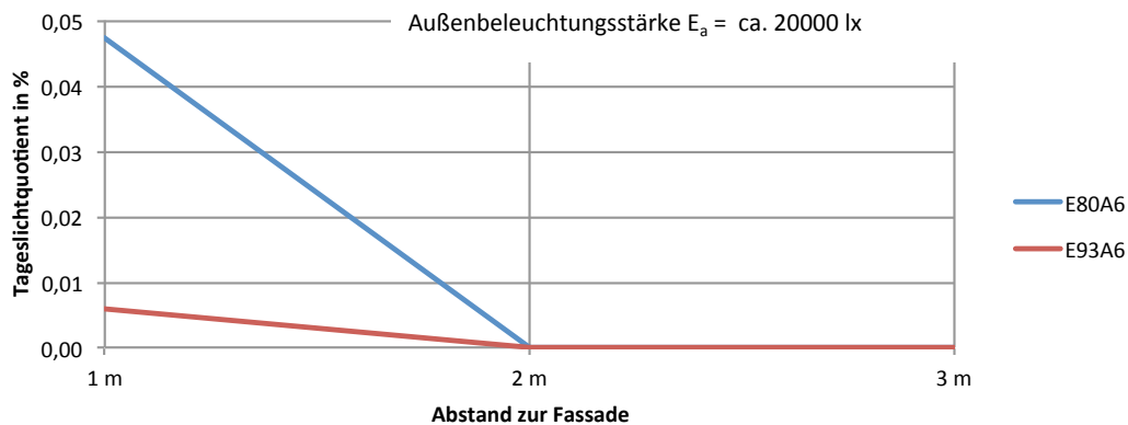
Tageslichtquotient Raffstoren E93A6 und E80A6 bei geschlossener Lamellenstellung
